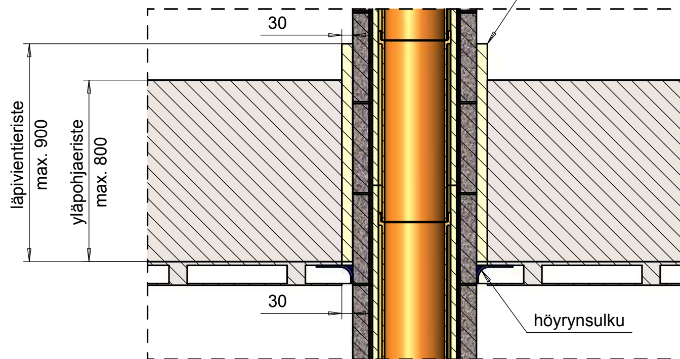
Yläpohjan läpivienti B 1:10
