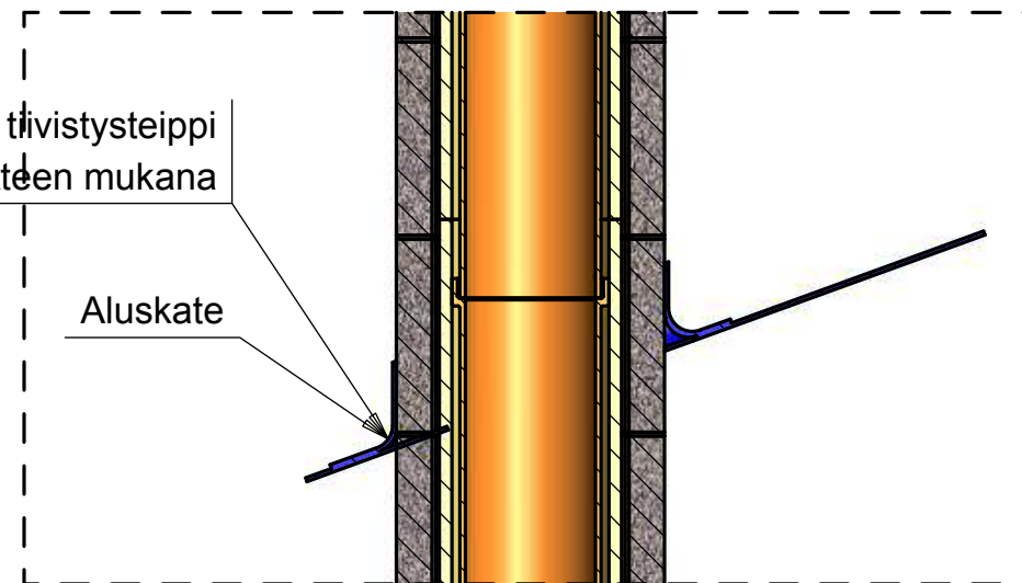
Vesikaton läpivienti A 1:10
